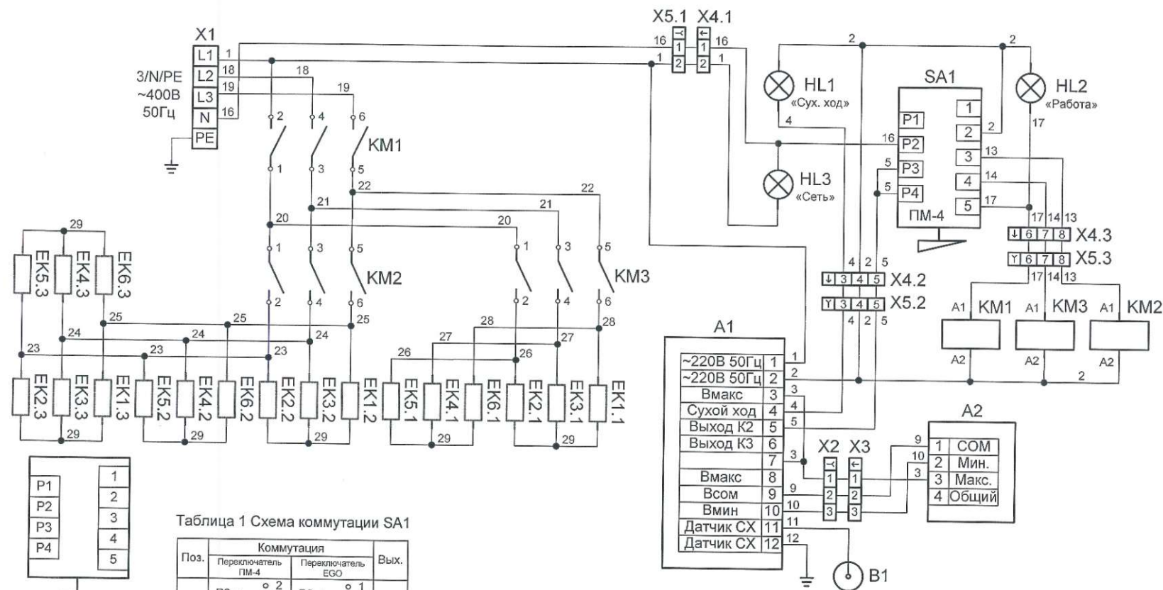
Рис.1 - Переключатель ПМ-4
