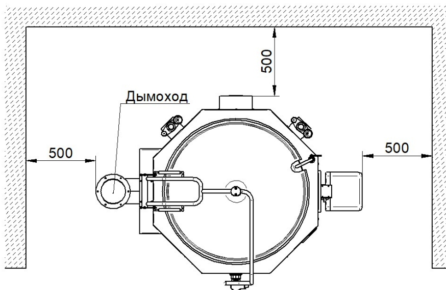
Рисунок 2 Установка котла
